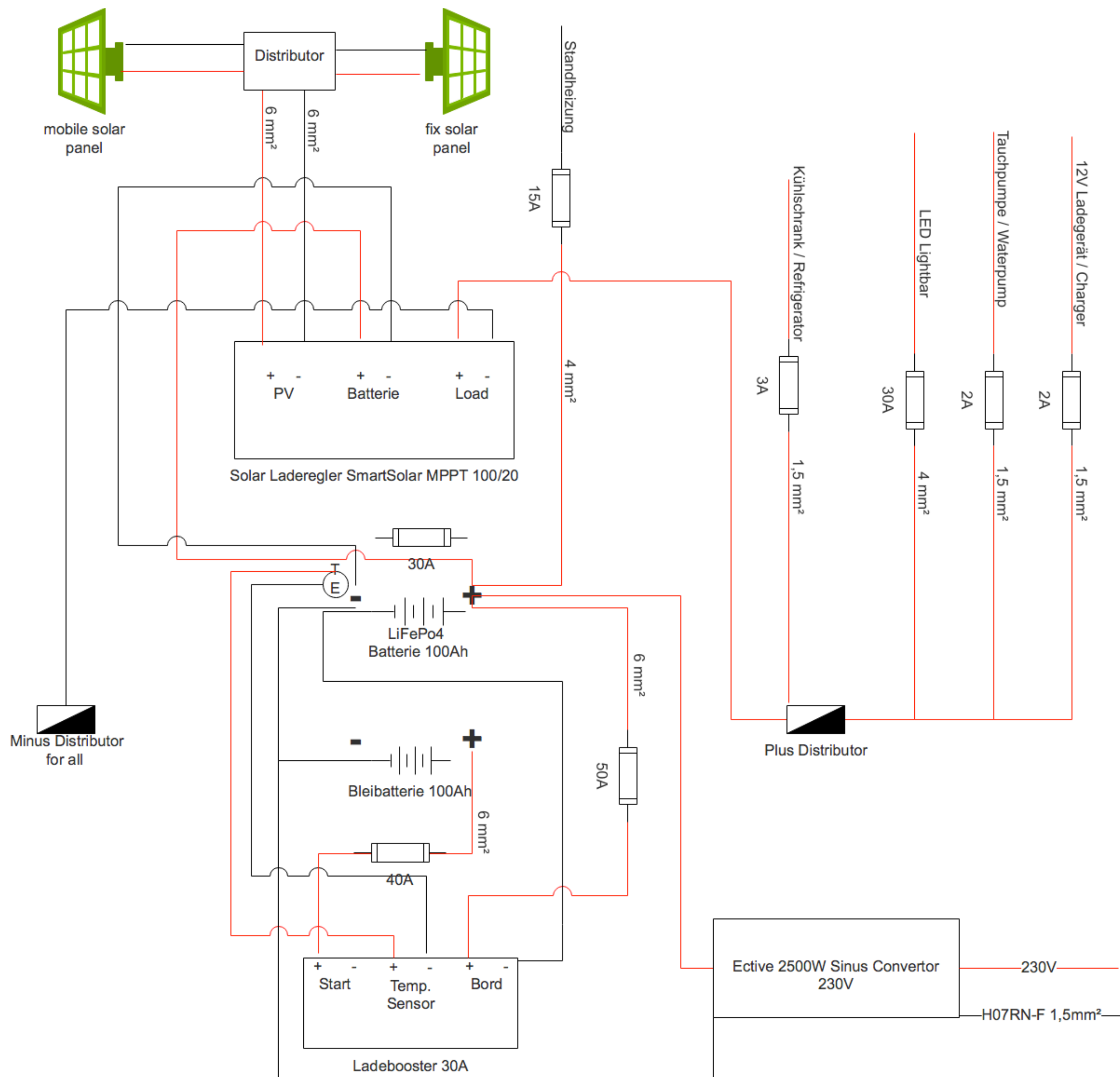
Elektroschaltplan - Pé na Estrada - Defender 110 Electric setup - Pé na Estrada - Defender 110
